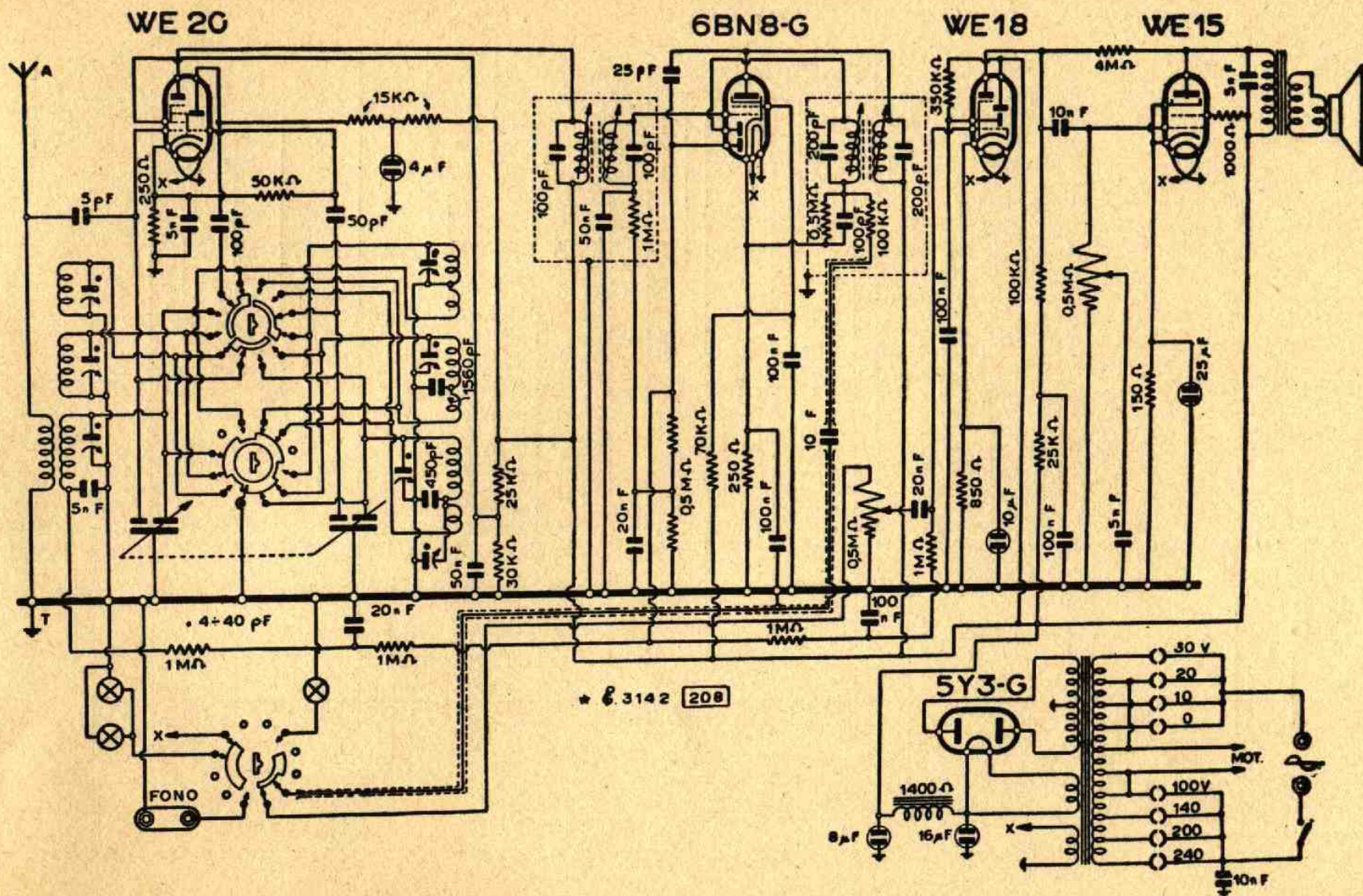
Lo schema elettrico del mod. "267,, Siare (telajo 2531)."
